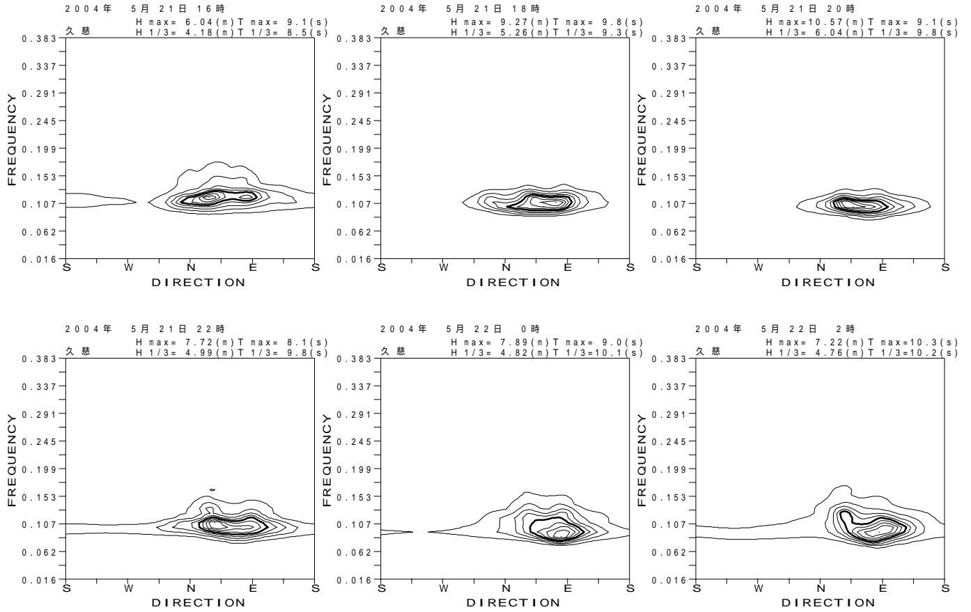
図 - 13.28 久慈 代表的な高波期間中の方向スペクトル
