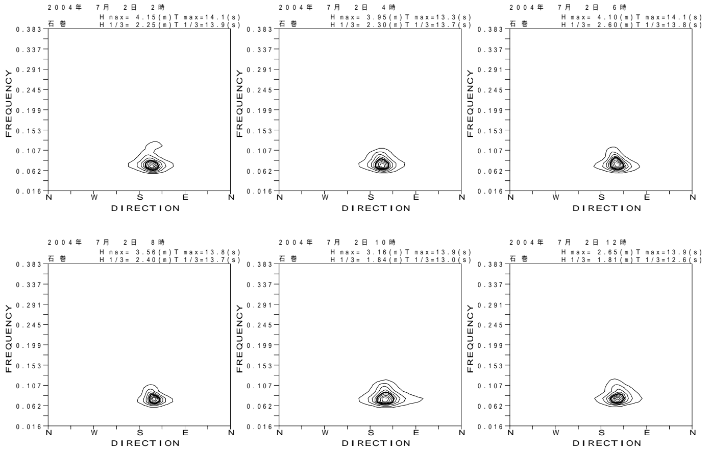
図 - 13.30 石巻 代表的な高波期間中の方向スペクトル
