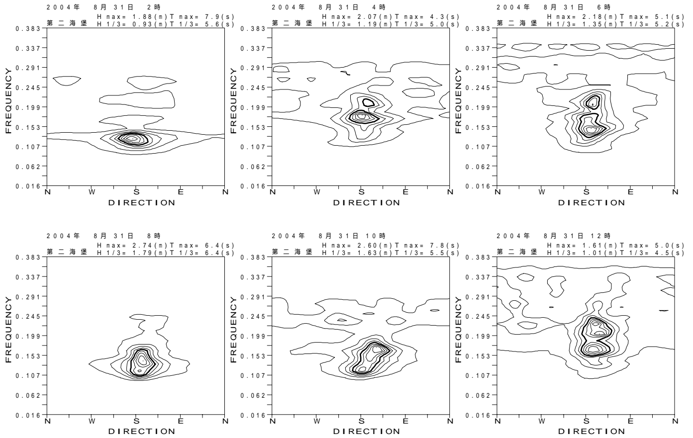
図 - 13.36 第二海堡 代表的な高波期間中の方向スペクトル
