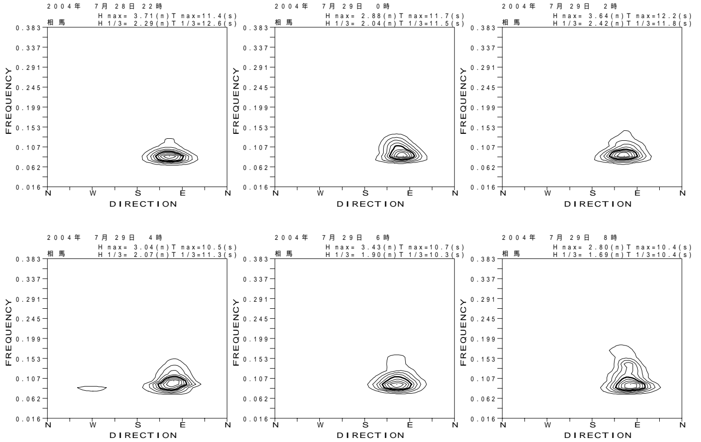
図 - 13.32 相馬 代表的な高波期間中の方向スペクトル
