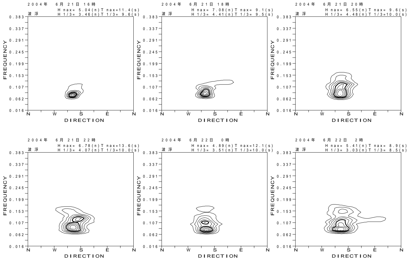
図 - 13.38 波浮 代表的な高波期間中の方向スペクトル
