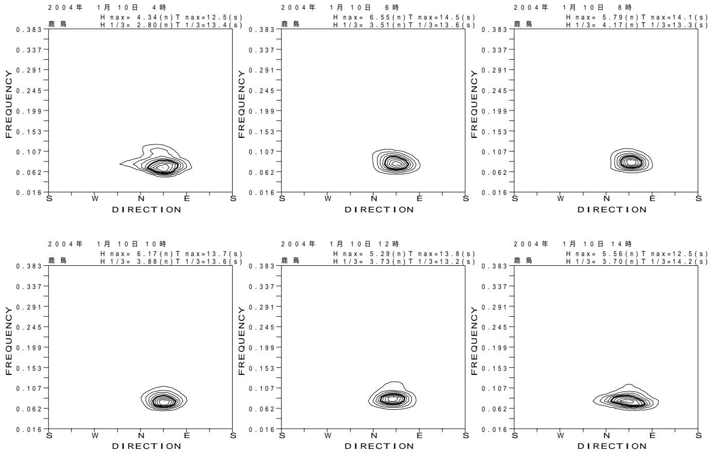
図 - 13.35 鹿島 代表的な高波期間中の方向スペクトル
