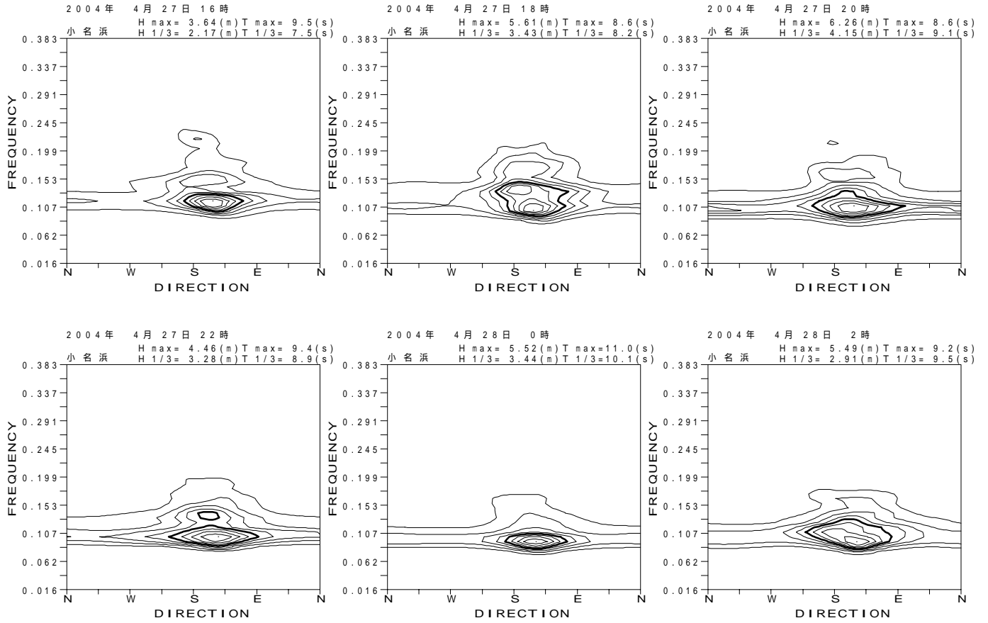
図 - 13.33 小名浜 代表的な高波期間中の方向スペクトル
