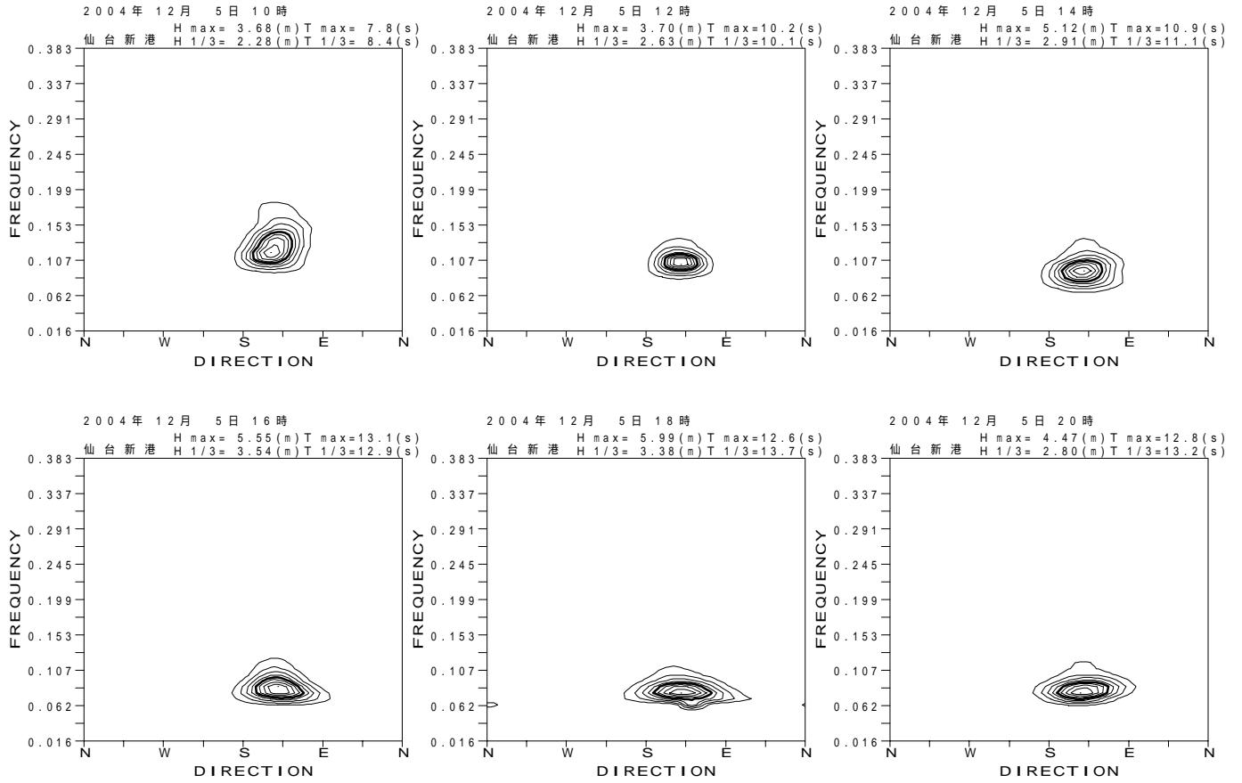
図 - 13.31 仙台新港 代表的な高波期間中の方向スペクトル
