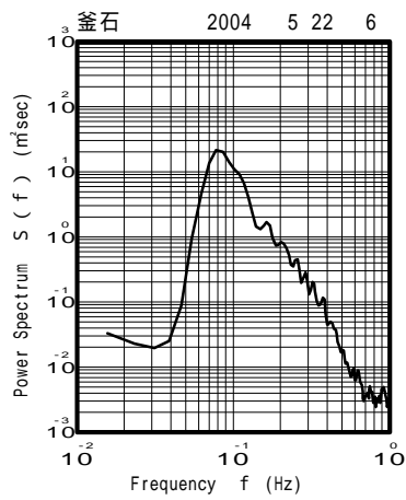
図 - 13.29 釜石 代表的な高波期間中のスペクトル
