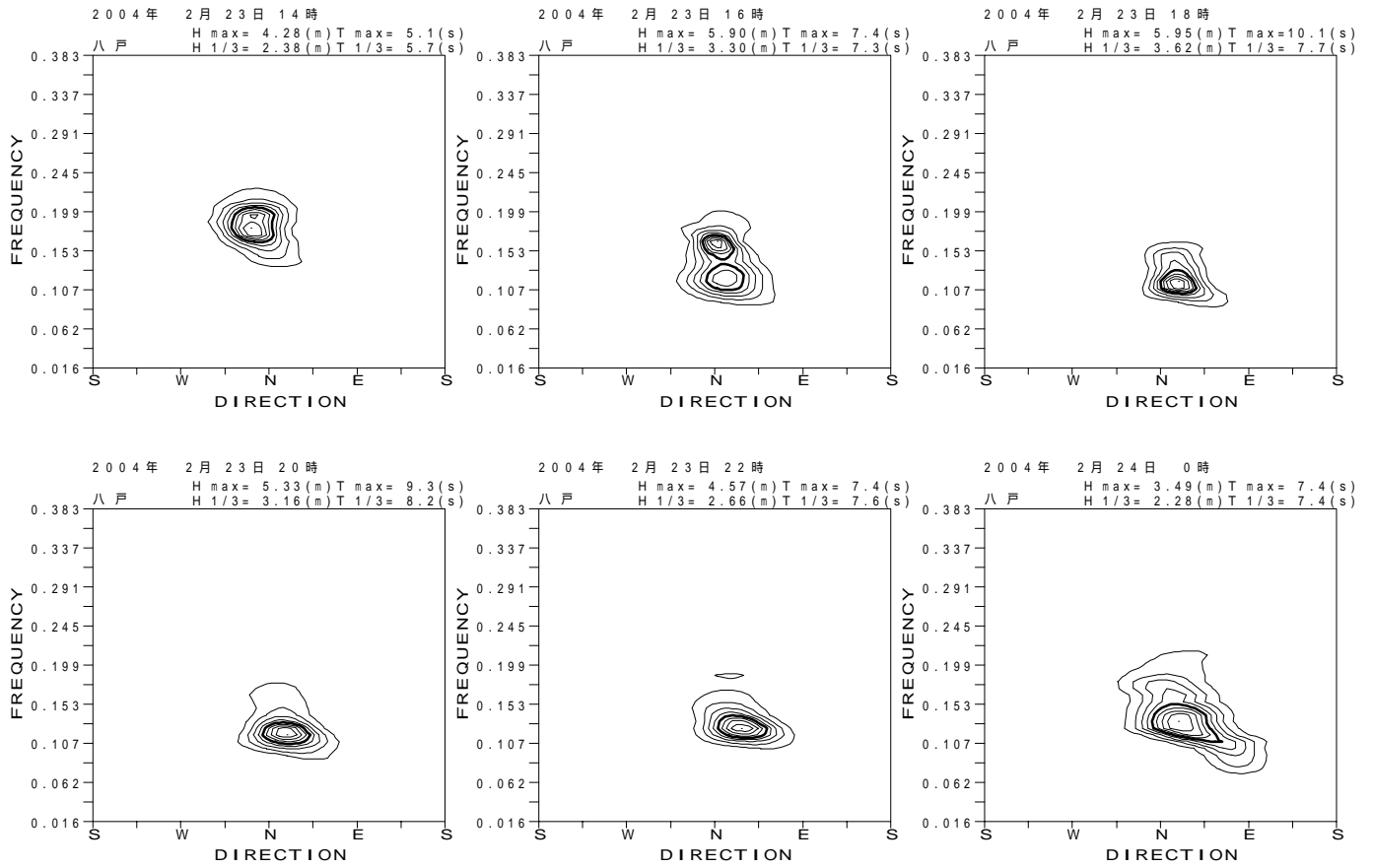
図 - 13.27 八戸 代表的な高波期間中の方向スペクトル
