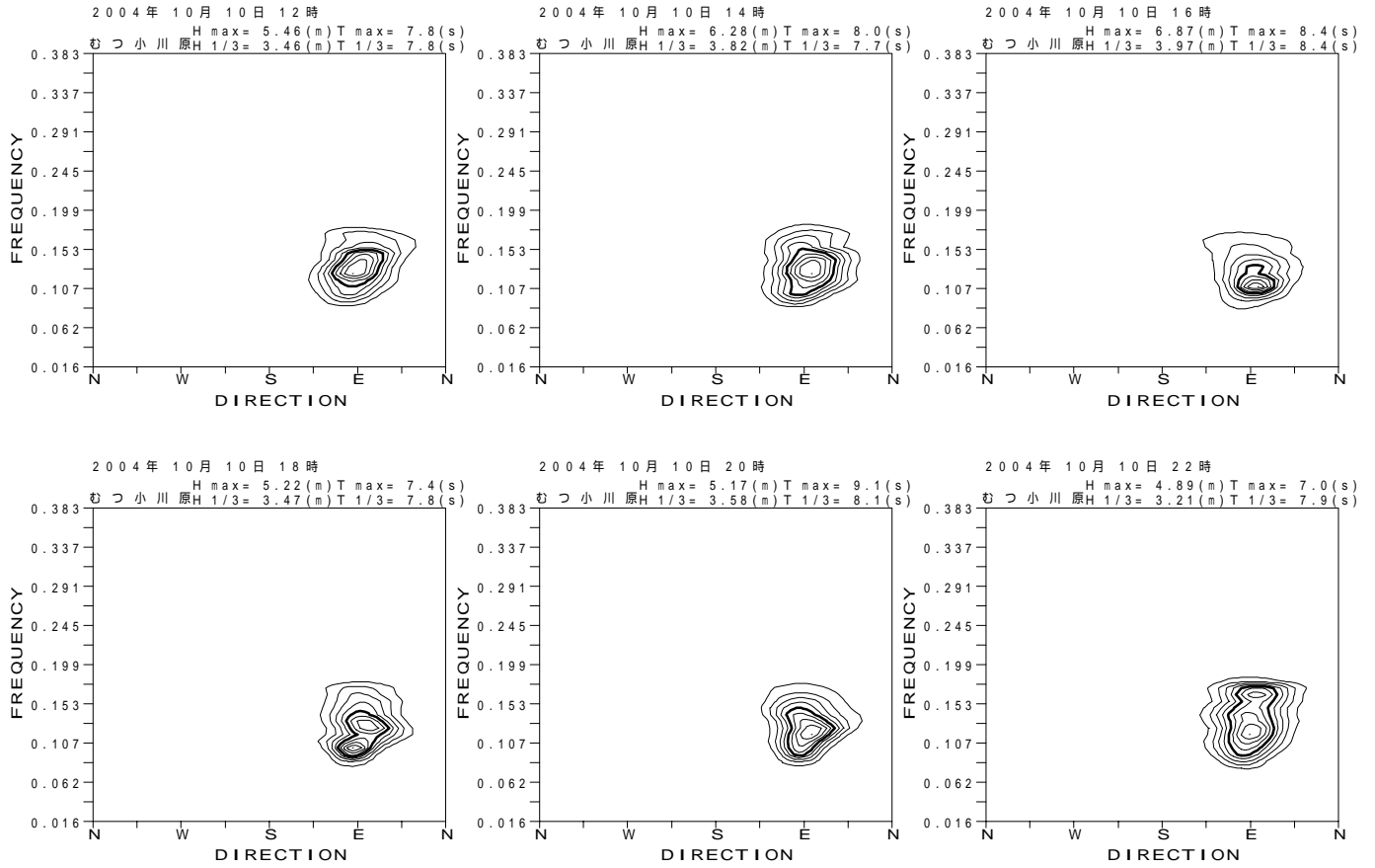
図 - 13.26 むつ小川原 代表的な高波期間中の方向スペクトル
