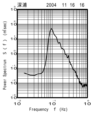
図 - 13.4 深浦 代表的な高波期間中のスペクトル
