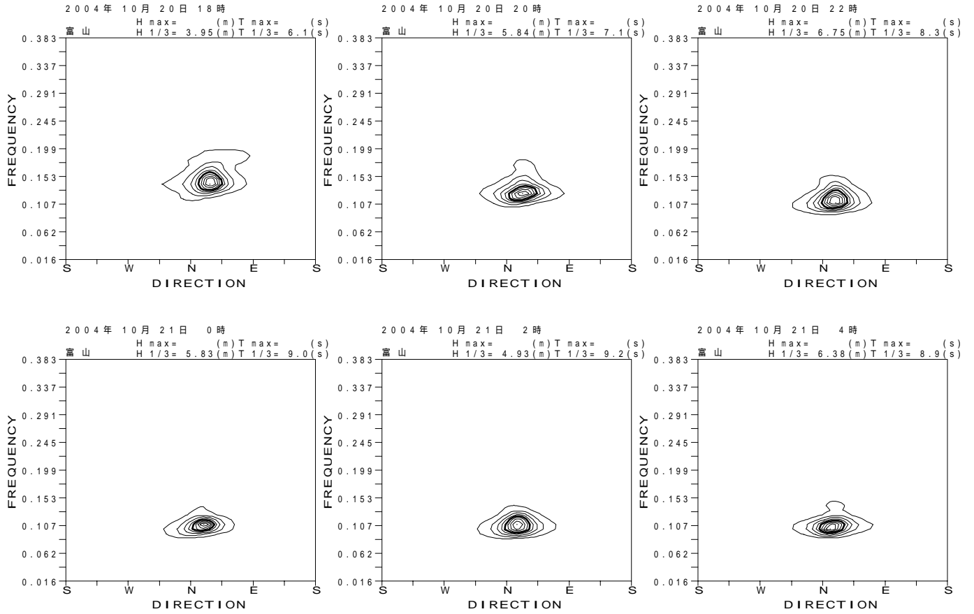
図 - 13.9 富山 代表的な高波期間中の方向スペクトル
