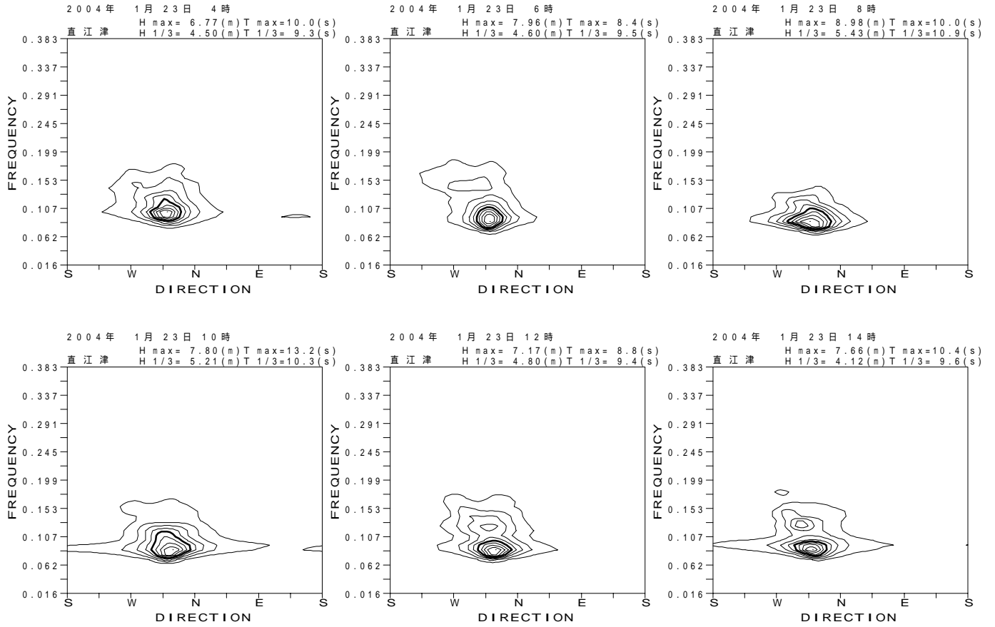
図 - 13.8 直江津 代表的な高波期間中の方向スペクトル
