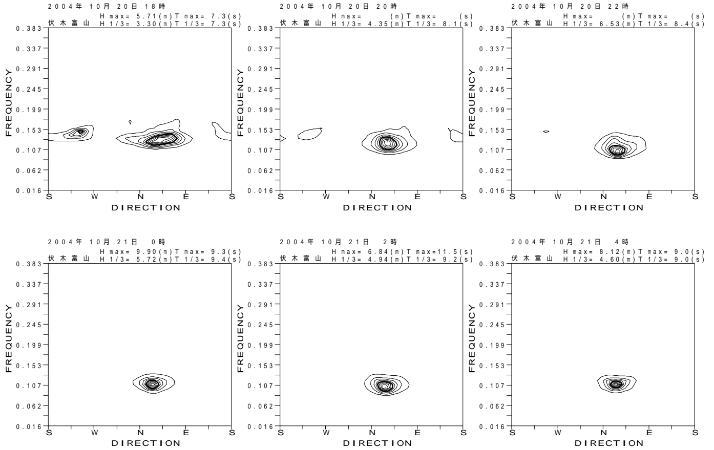
図 - 13.10 伏木富山 代表的な高波期間中の方向スペクトル
