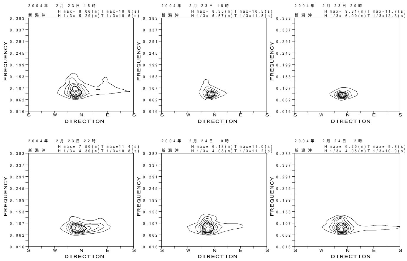
図 - 13.7 新潟沖 代表的な高波期間中の方向スペクトル
