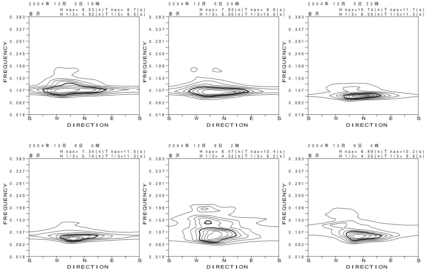
図 - 13.12 金沢 代表的な高波期間中の方向スペクトル
