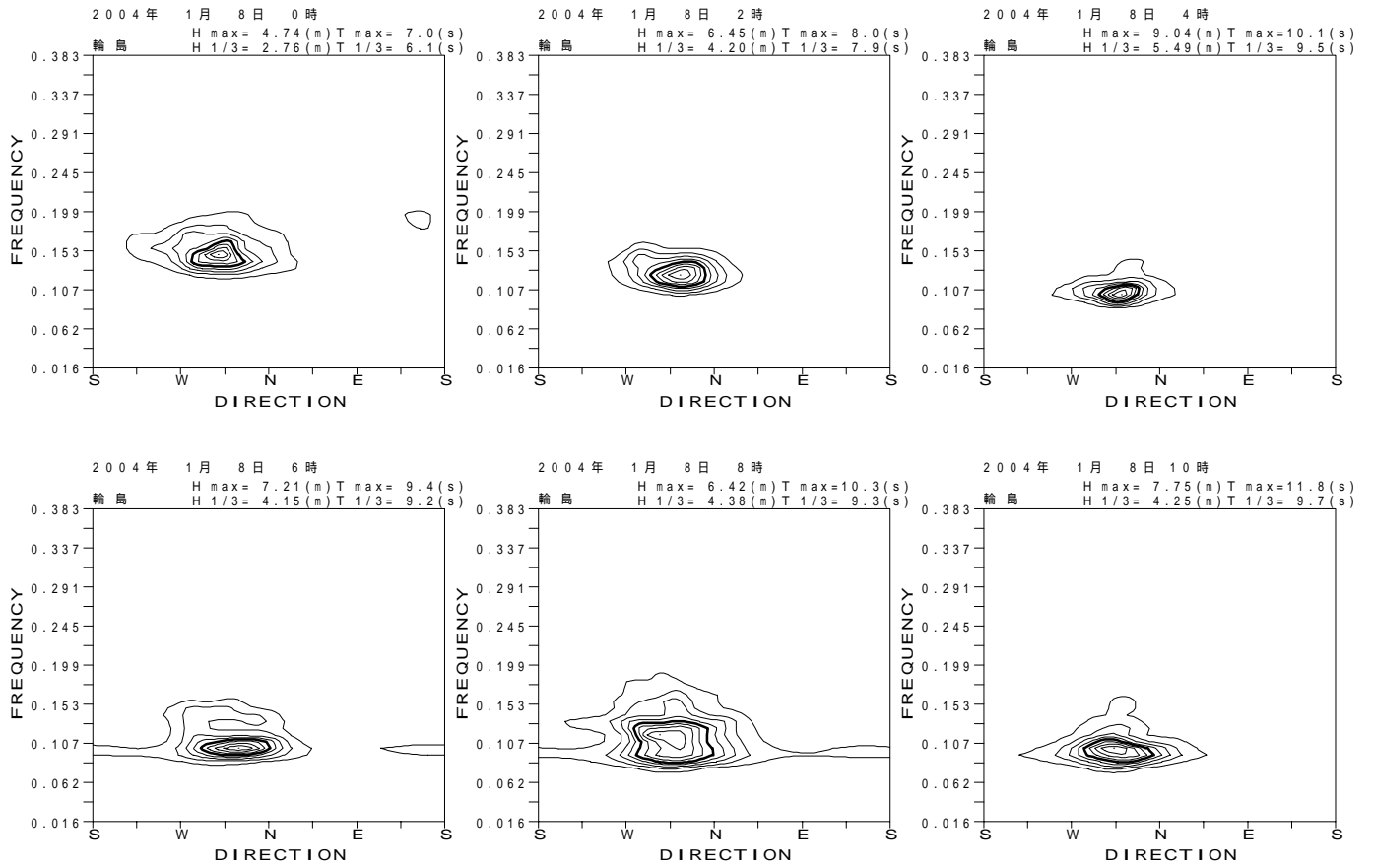
図 - 13.11 輪島 代表的な高波期間中の方向スペクトル
