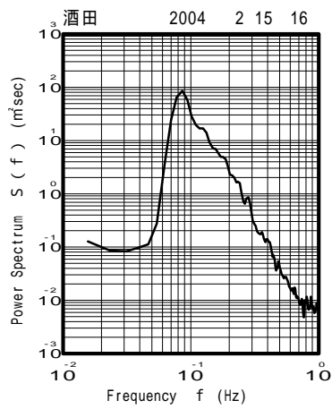
図 - 13.6 酒田 代表的な高波期間中のスペクトル
