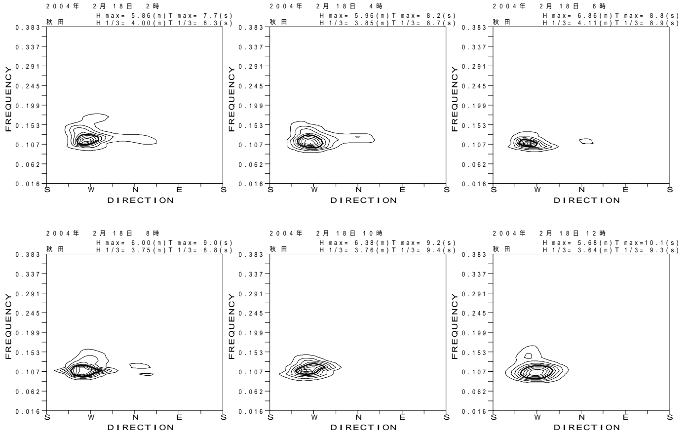
図 - 13.5 秋田 代表的な高波期間中の方向スペクトル
