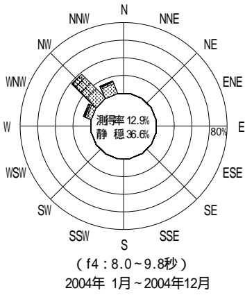
図 - 12.2 石狩新港 波高・波向別出現頻度図 ( f2 , f3 , f4 , f5 , 全周期帯 )
