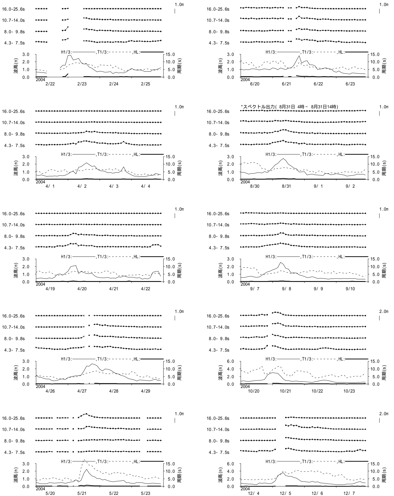
図 - 11.37 アシカ島 周期帯別波浪特性の経時変化(高波期間中)
