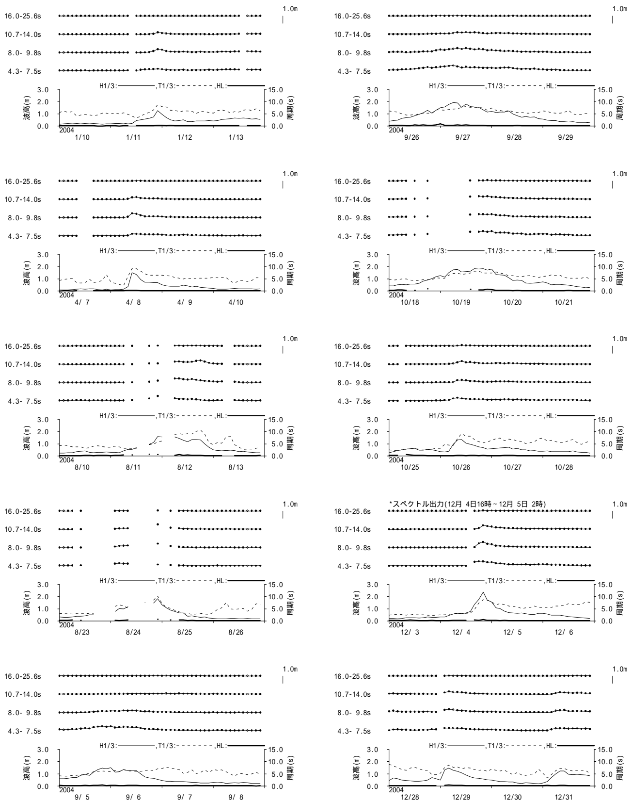
図 - 11.56 石垣 周期帯別波浪特性の経時変化(高波期間中)
