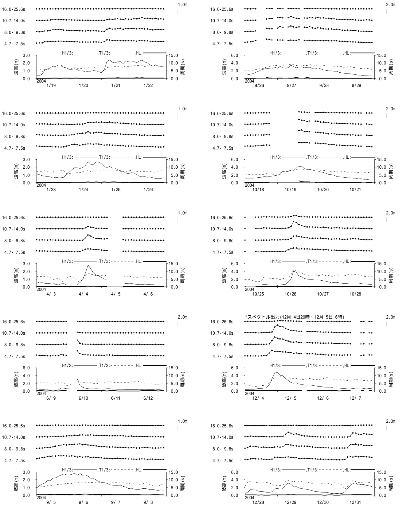
図 - 11.55 平良 周期帯別波浪特性の経時変化(高波期間中)
