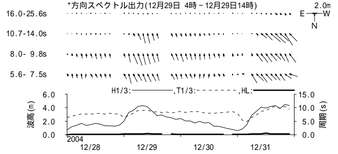
図 - 11.22 那覇 周期帯別波浪特性の経時変化(高波期間中)
