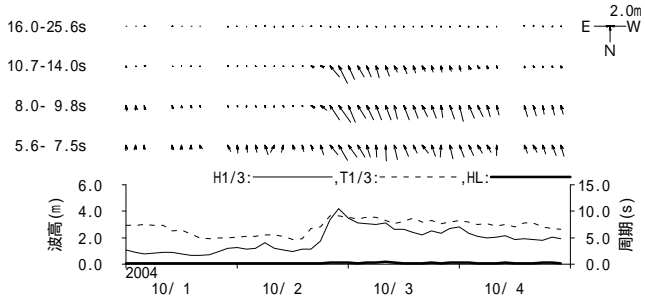
図 - 11.22 那覇 周期帯別波浪特性の経時変化(高波期間中)
