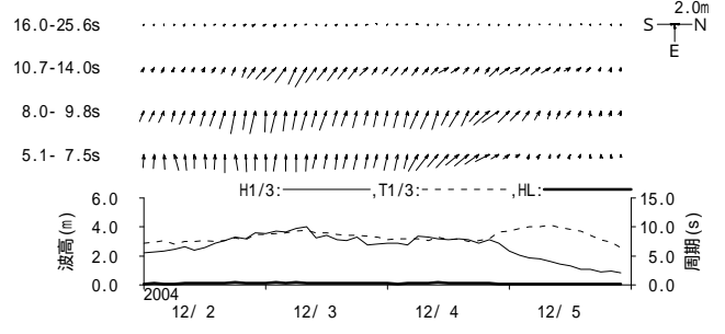
図 - 11.54 中城湾 周期帯別波浪特性の経時変化(高波期間中)
