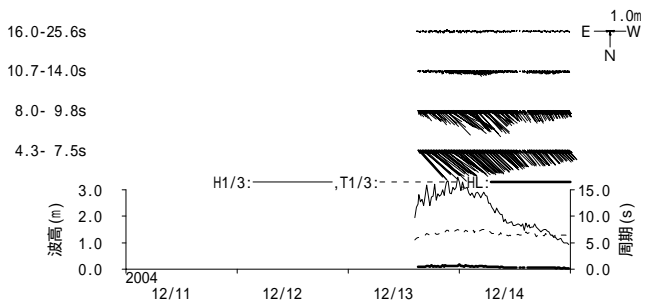
図 - 11.2 石狩新港 周期帯別波浪特性の経時変化(高波期間中)
