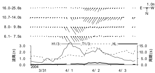
図 - 11.23 紋別(南) 周期帯別波浪特性の経時変化(高波期間中)
