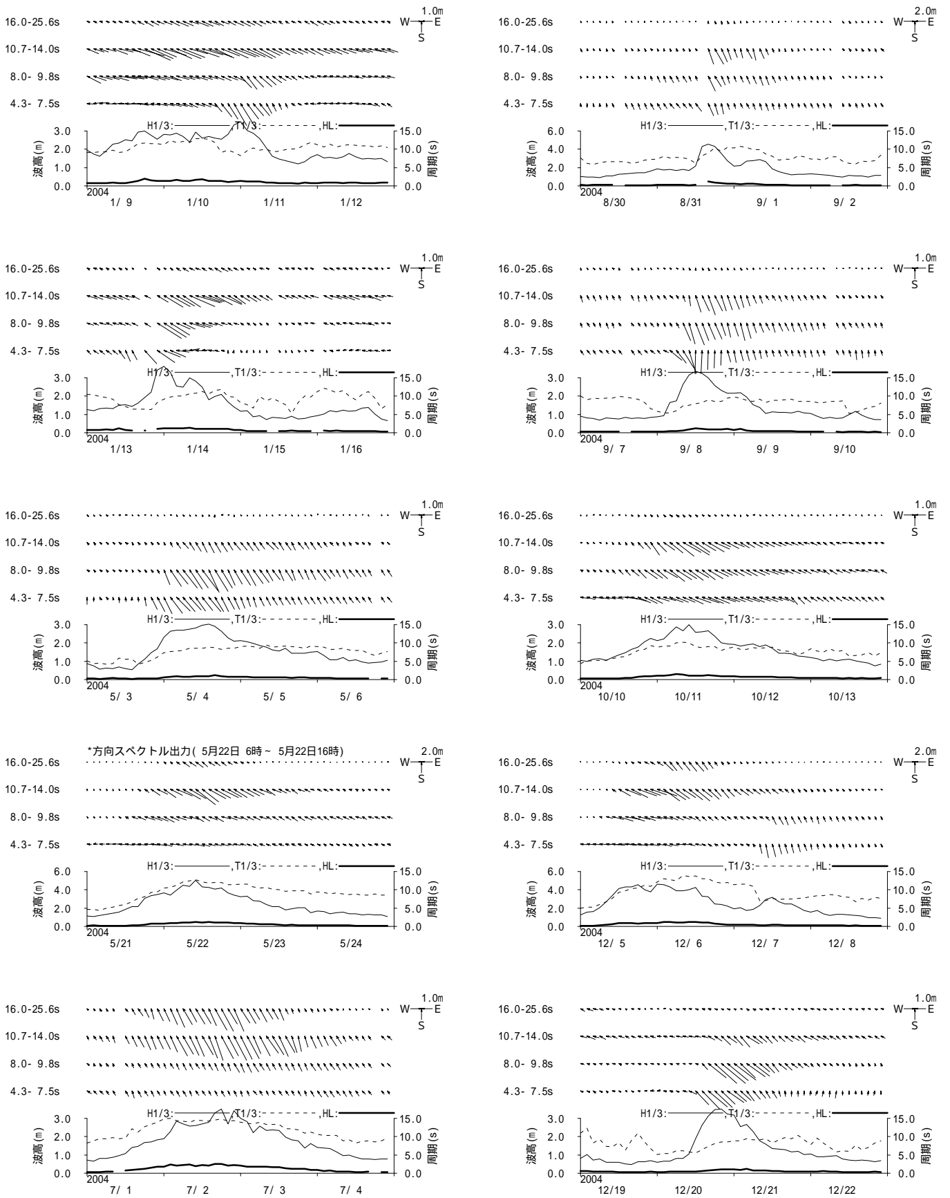
図 - 11.24 十勝 周期帯別波浪特性の経時変化(高波期間中)
