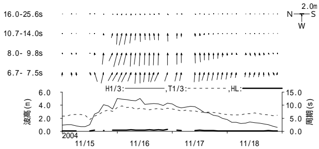
図 - 11.3 瀬棚 周期帯別波浪特性の経時変化(高波期間中)
