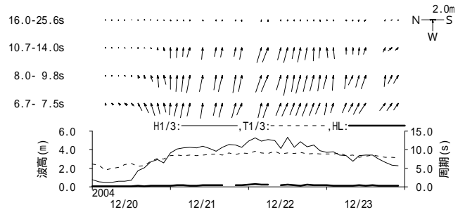
図 - 11.3 瀬棚 周期帯別波浪特性の経時変化(高波期間中)
