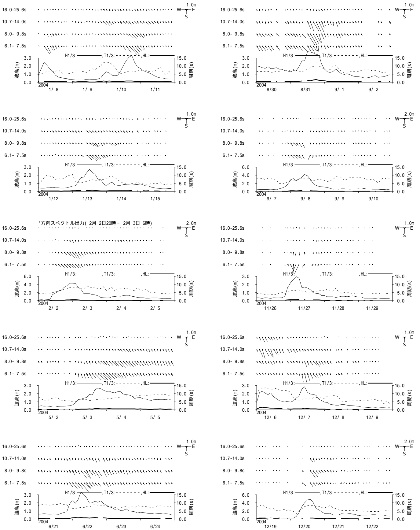
図 - 11.25 苫小牧 周期帯別波浪特性の経時変化(高波期間中)
