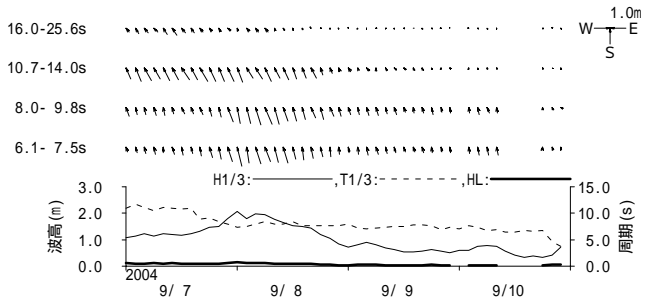
図 - 11.40 清水 周期帯別波浪特性の経時変化(高波期間中)
