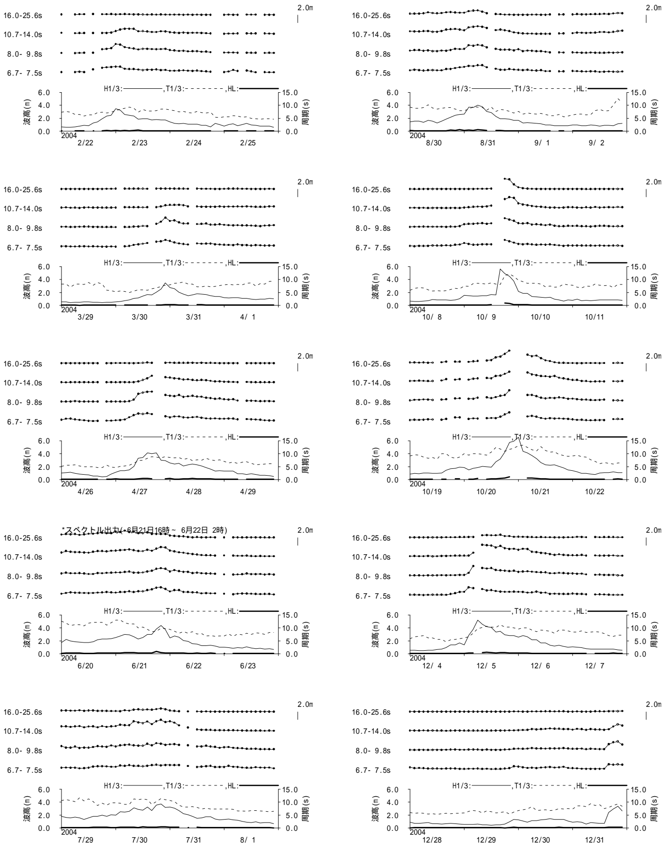
図 - 11.39 下田 周期帯別波浪特性の経時変化(高波期間中)
