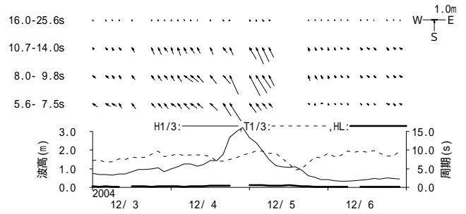
図 - 11.52 志布志湾 周期帯別波浪特性の経時変化(高波期間中)
