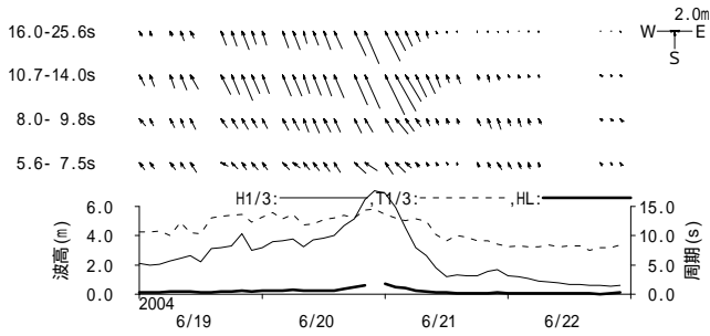
図 - 11.52 志布志湾 周期帯別波浪特性の経時変化(高波期間中)
