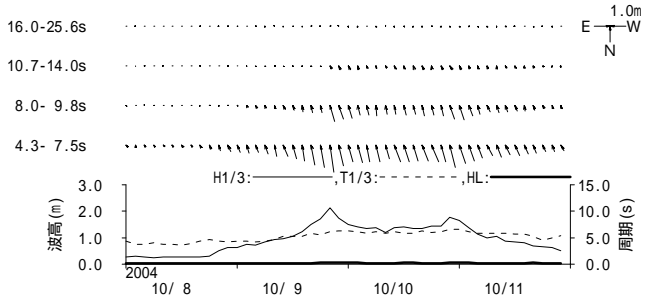
図 - 11.18 藍島 周期帯別波浪特性の経時変化(高波期間中)
