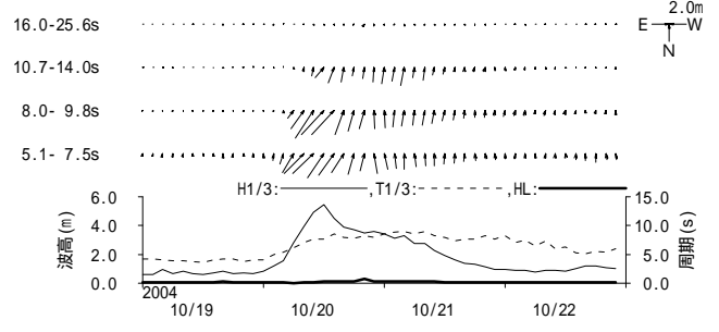
図 - 11.19 玄界灘 周期帯別波浪特性の経時変化(高波期間中)
