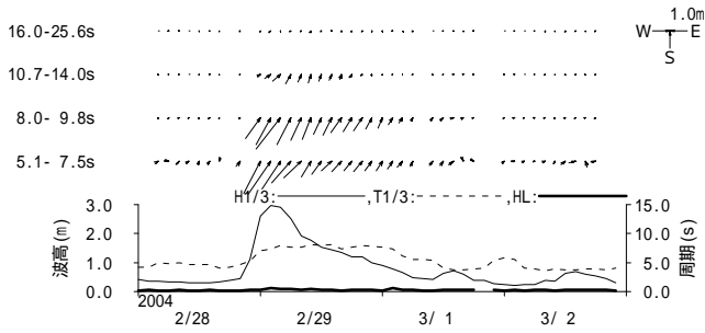
図 - 11.20 伊王島 周期帯別波浪特性の経時変化(高波期間中)
