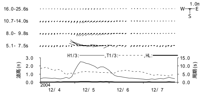
図 - 11.20 伊王島 周期帯別波浪特性の経時変化(高波期間中)
