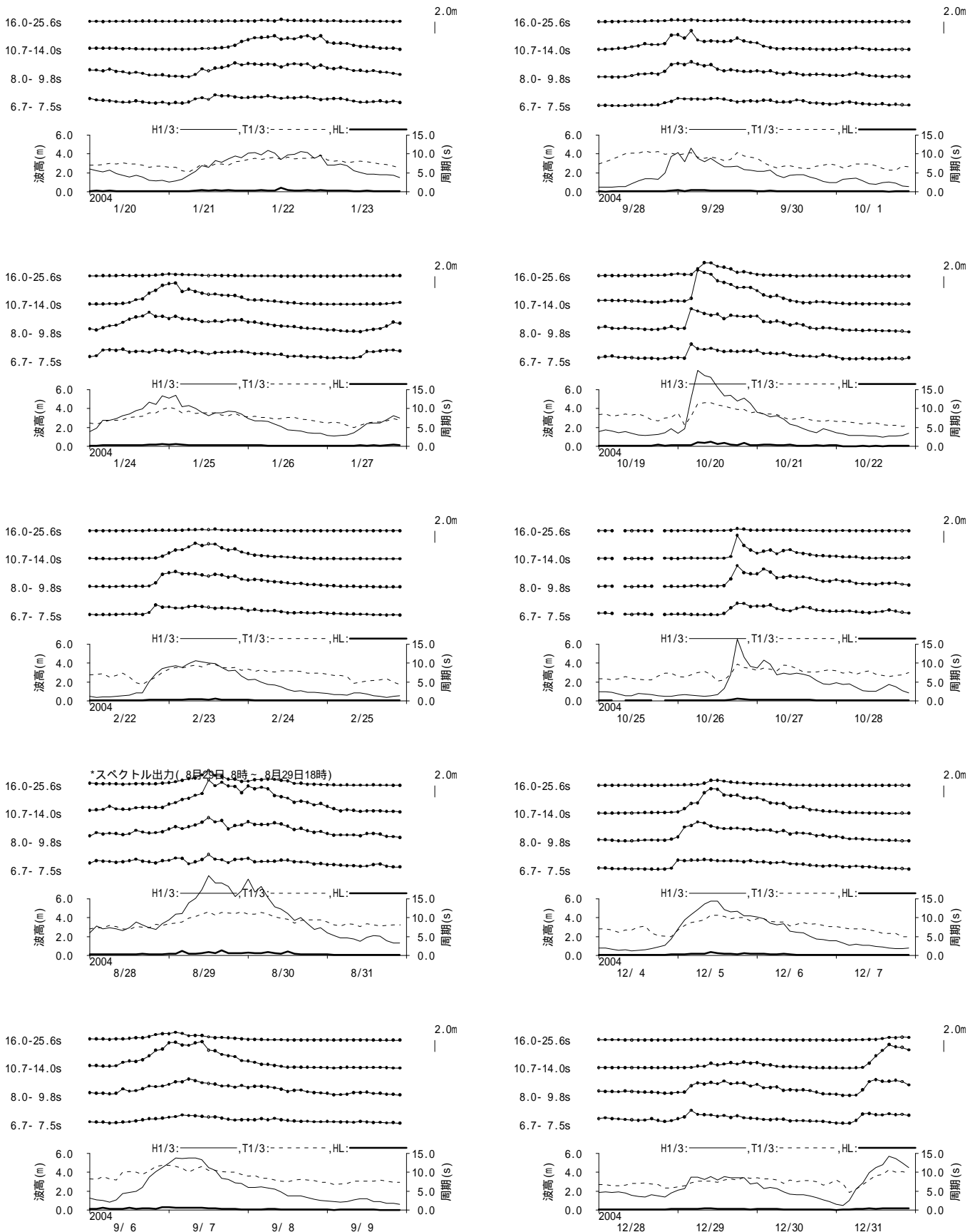
図 - 11.21 名瀬 周期帯別波浪特性の経時変化(高波期間中)
