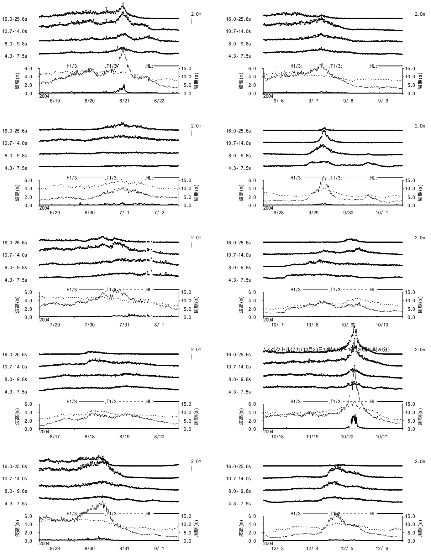
図 - 11.46 室戸GPS 周期帯別波浪特性の経時変化(高波期間中)
