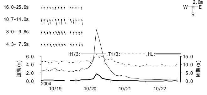
図 - 11.48 高知 周期帯別波浪特性の経時変化(高波期間中)
