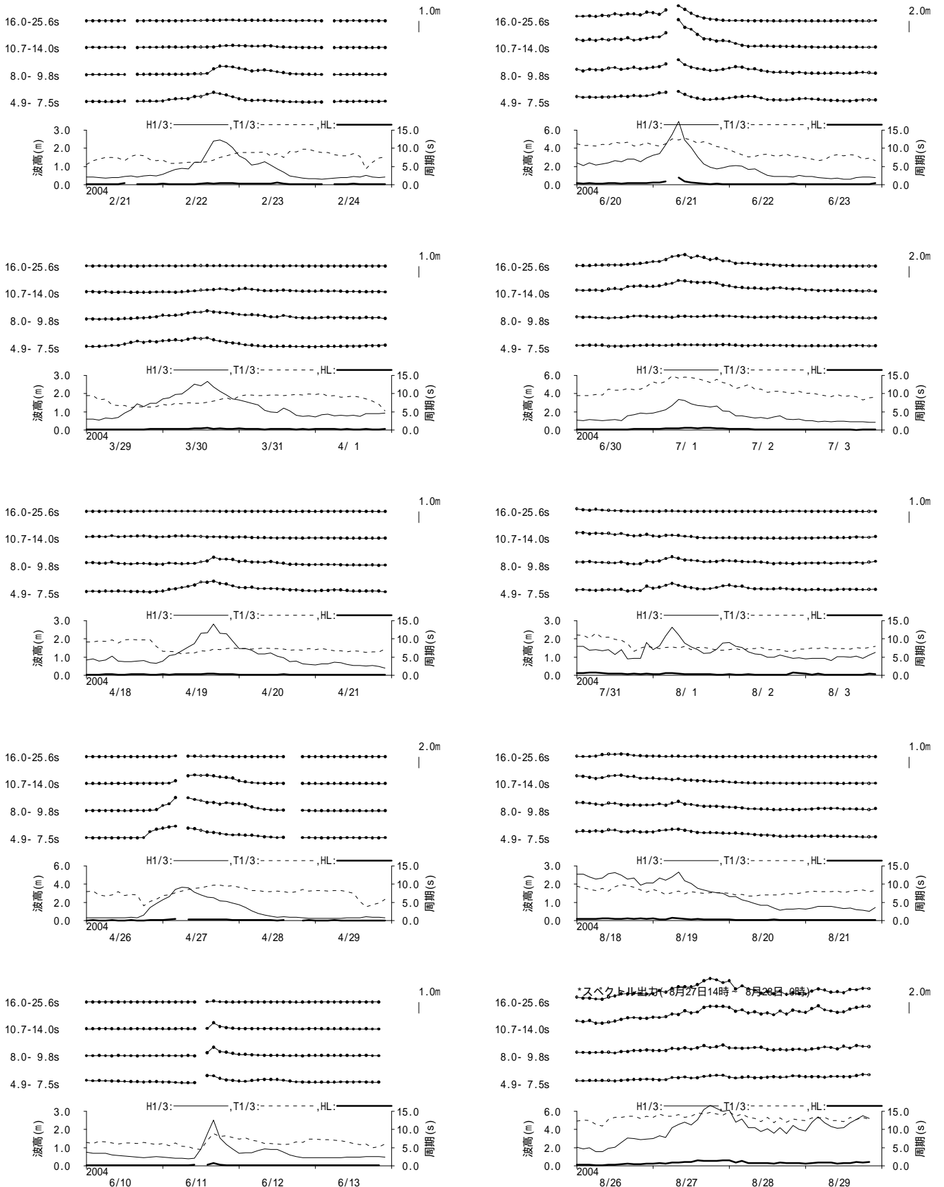
図 - 11.49 上川口 周期帯別波浪特性の経時変化(高波期間中)
