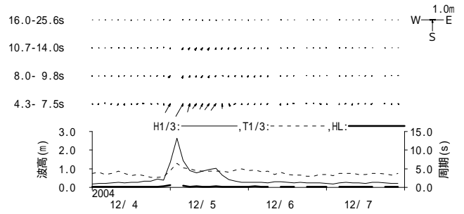
図 - 11.44 神戸 周期帯別波浪特性の経時変化(高波期間中)
