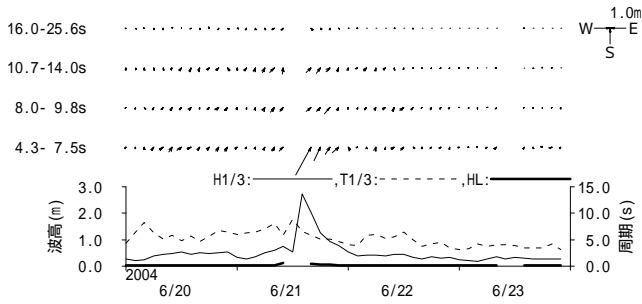
図 - 11.44 神戸 周期帯別波浪特性の経時変化(高波期間中)
