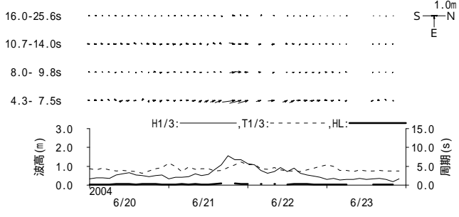
図 - 11.36 第二海堡 周期帯別波浪特性の経時変化(高波期間中)
