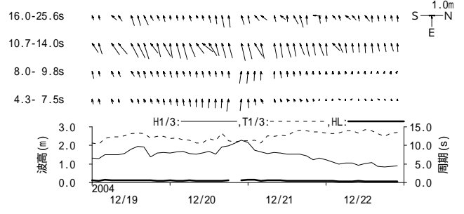
図 - 11.32 相馬 周期帯別波浪特性の経時変化(高波期間中)
