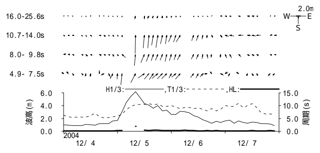
図 - 11.38 波浮 周期帯別波浪特性の経時変化(高波期間中)
