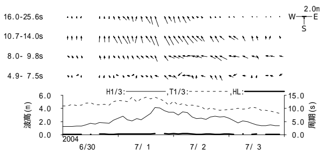
図 - 11.38 波浮 周期帯別波浪特性の経時変化(高波期間中)
