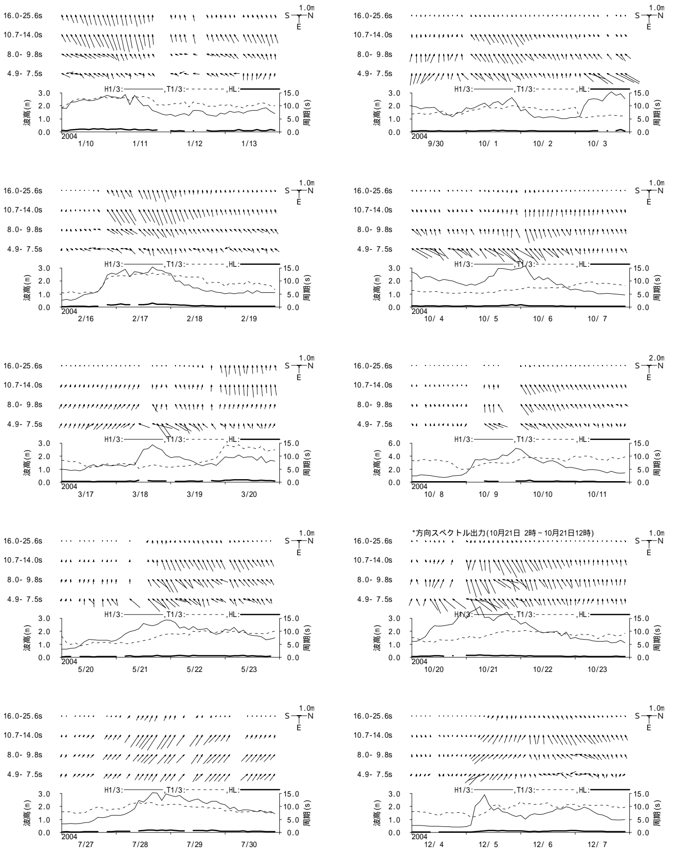
図 - 11.34 常陸那珂 周期帯別波浪特性の経時変化(高波期間中)
