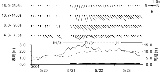
図 - 11.35 鹿島 周期帯別波浪特性の経時変化(高波期間中)
