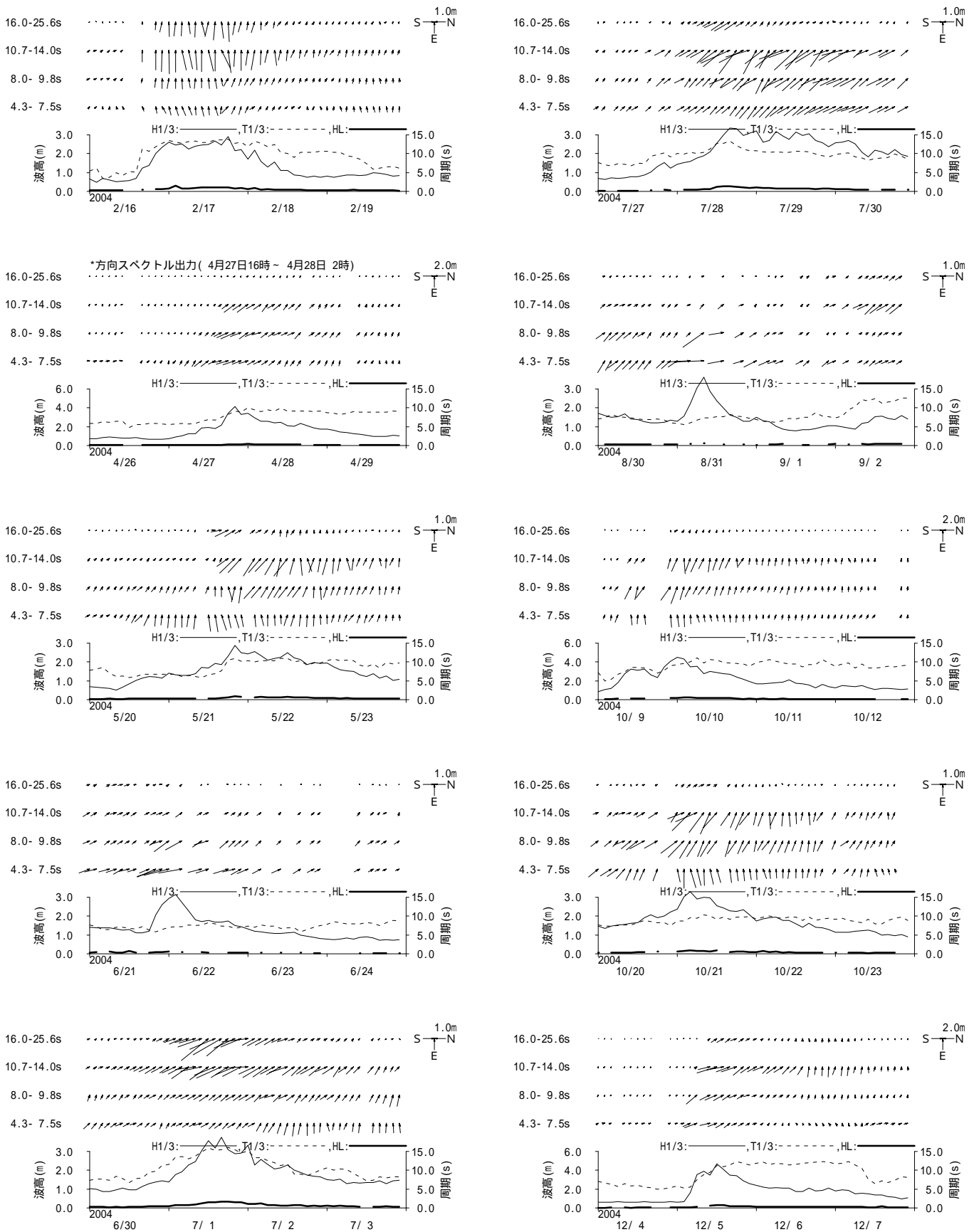
図 - 11.33 小名浜 周期帯別波浪特性の経時変化(高波期間中)
