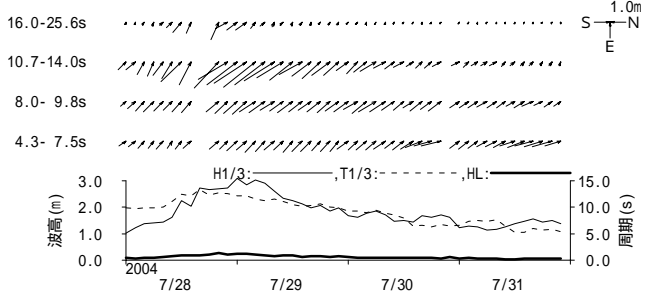
図 - 11.31 仙台新港 周期帯別波浪特性の経時変化(高波期間中)
