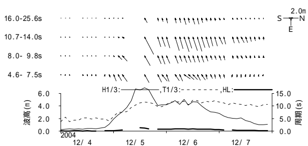
図 - 11.27 八戸 周期帯別波浪特性の経時変化(高波期間中)
